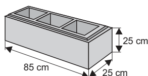
Bloczek podmurówkowy
