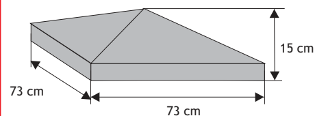
Daszek słupkowy do poddasza grubego (bez okapnika)
