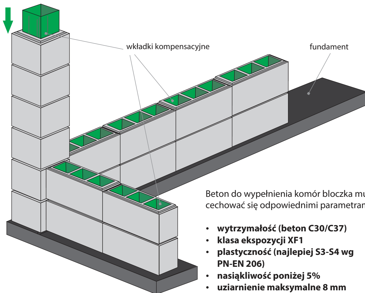
Rys. Stosowanie wkładek kompensacyjnych.
