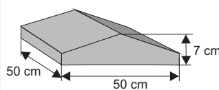
Daszek słupkowy do poddasza cienkiego dwuspadowy (z półokapnikiem)
