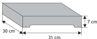
Daszek systemowy płaski (wystający) z pełnym okapnikiem
