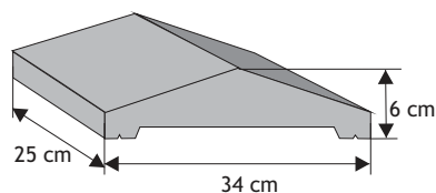
Daszek systemowy dwuspadowy (wystający) z pełnym okapnikiem
