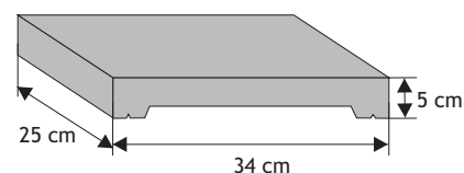
Daszek systemowy płaski (wystający) z pełnym okapnikiem
