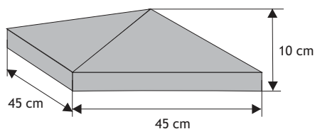
Daszek koperta (z półokapnikiem)
