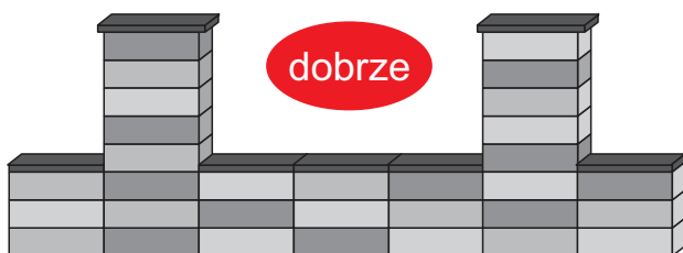
Rys. Montaż i klejenie bloczków.
