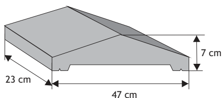
Daszek dwuspadowy (z pełnym okapnikiem)
