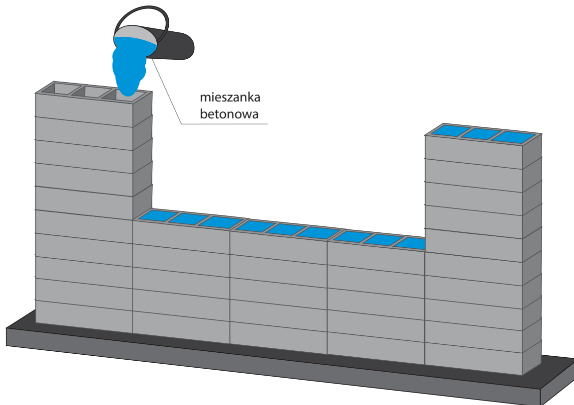
Rys. Wypełnianie bloczków mieszanką betonową.
