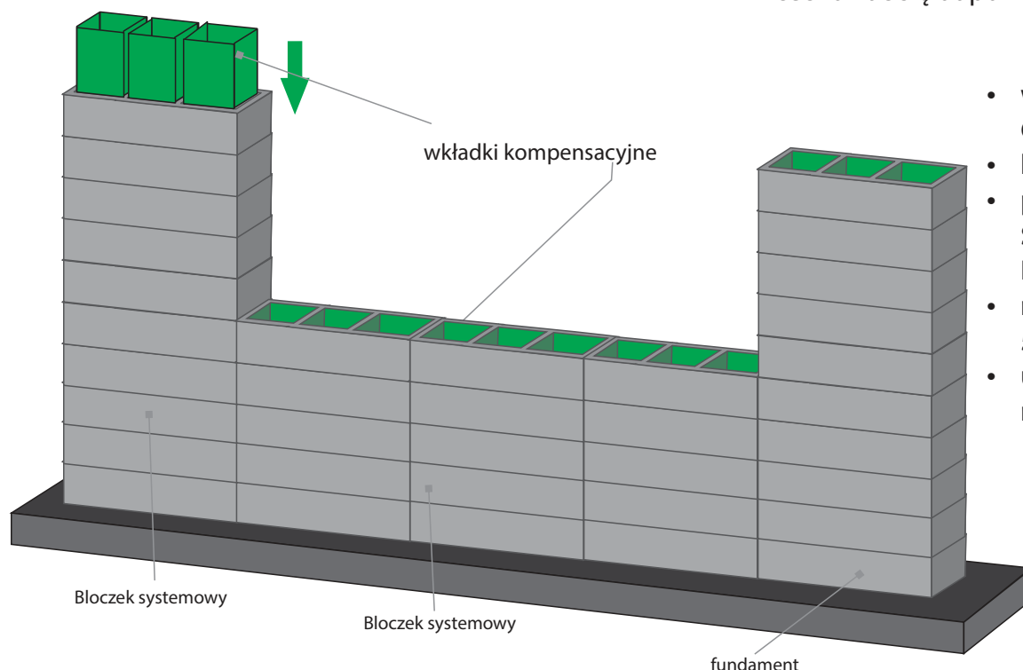
Rys. Stosowanie wkładek kompensacyjnych.
