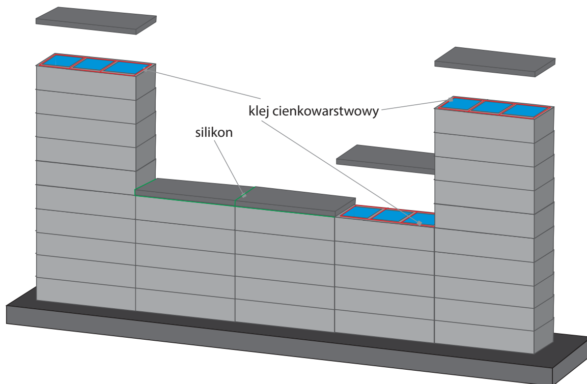
Rys. Montaż daszków.
