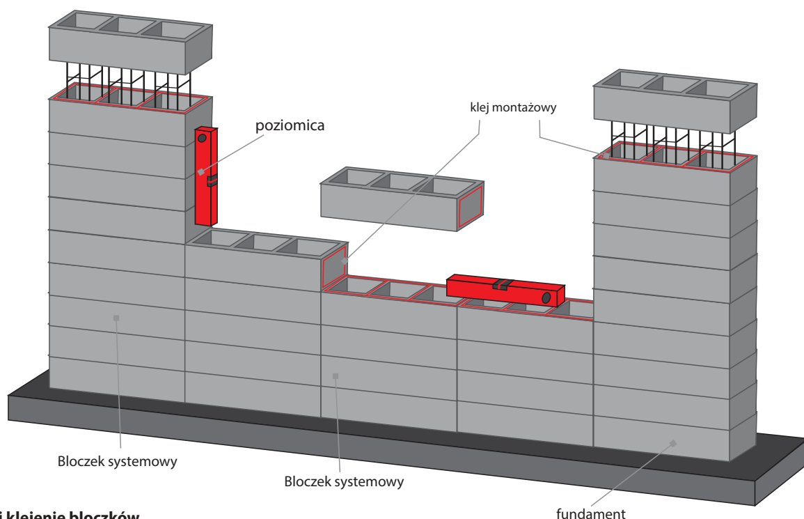
Rys. Montaż i klejenie bloczków.
