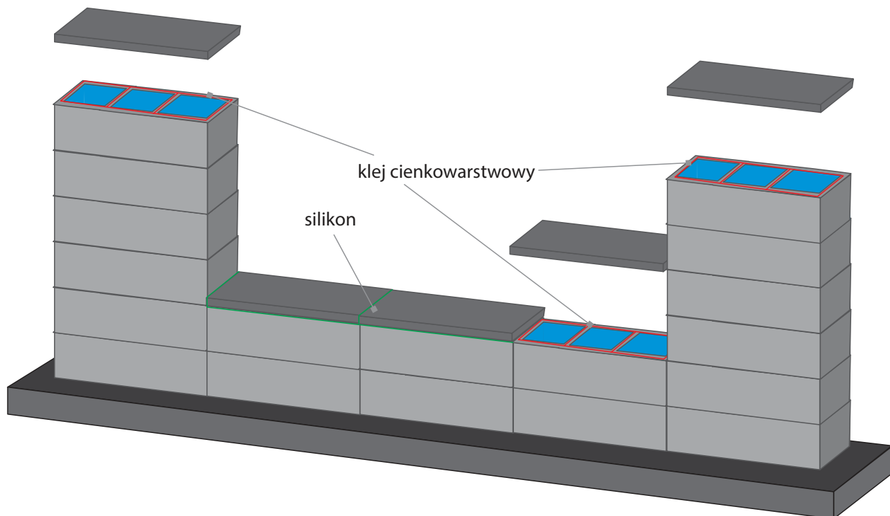
Rys. Montaż daszków.
