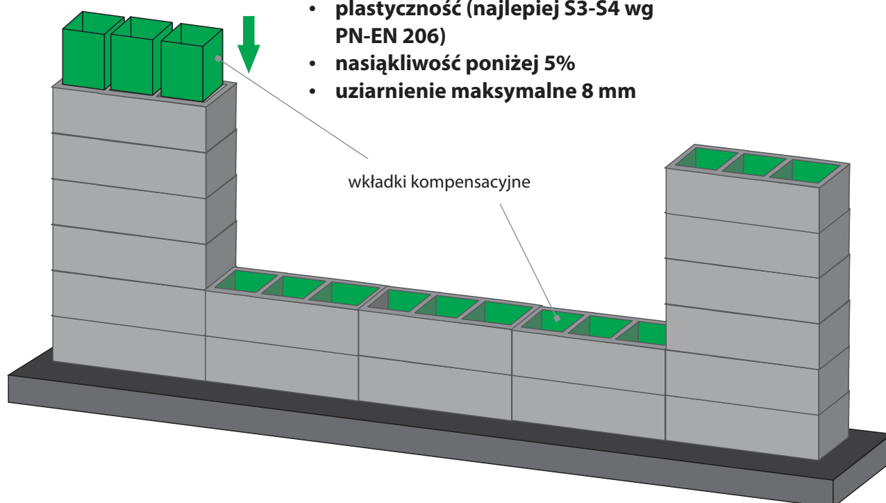
Rys. Stosowanie wkładek kompensacyjnych.
